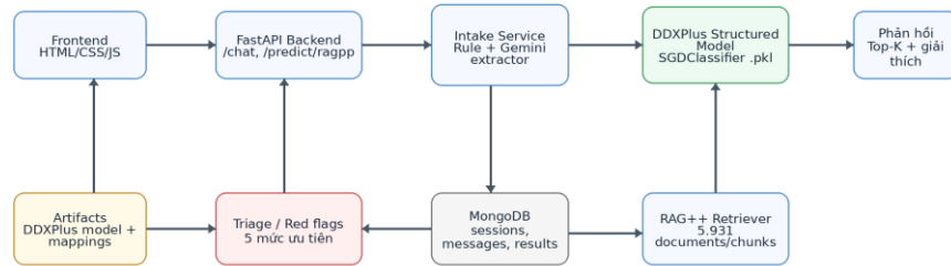
Kiến trúc tổng quan Healthcare Chatbot DDXPlus không train tiếng Việt
